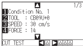
Anzeige CONDITION (Normal-Modus)
